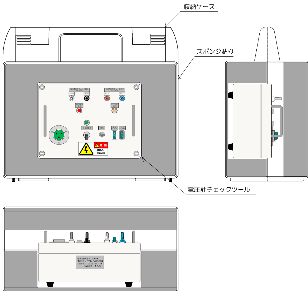
収納概略図
